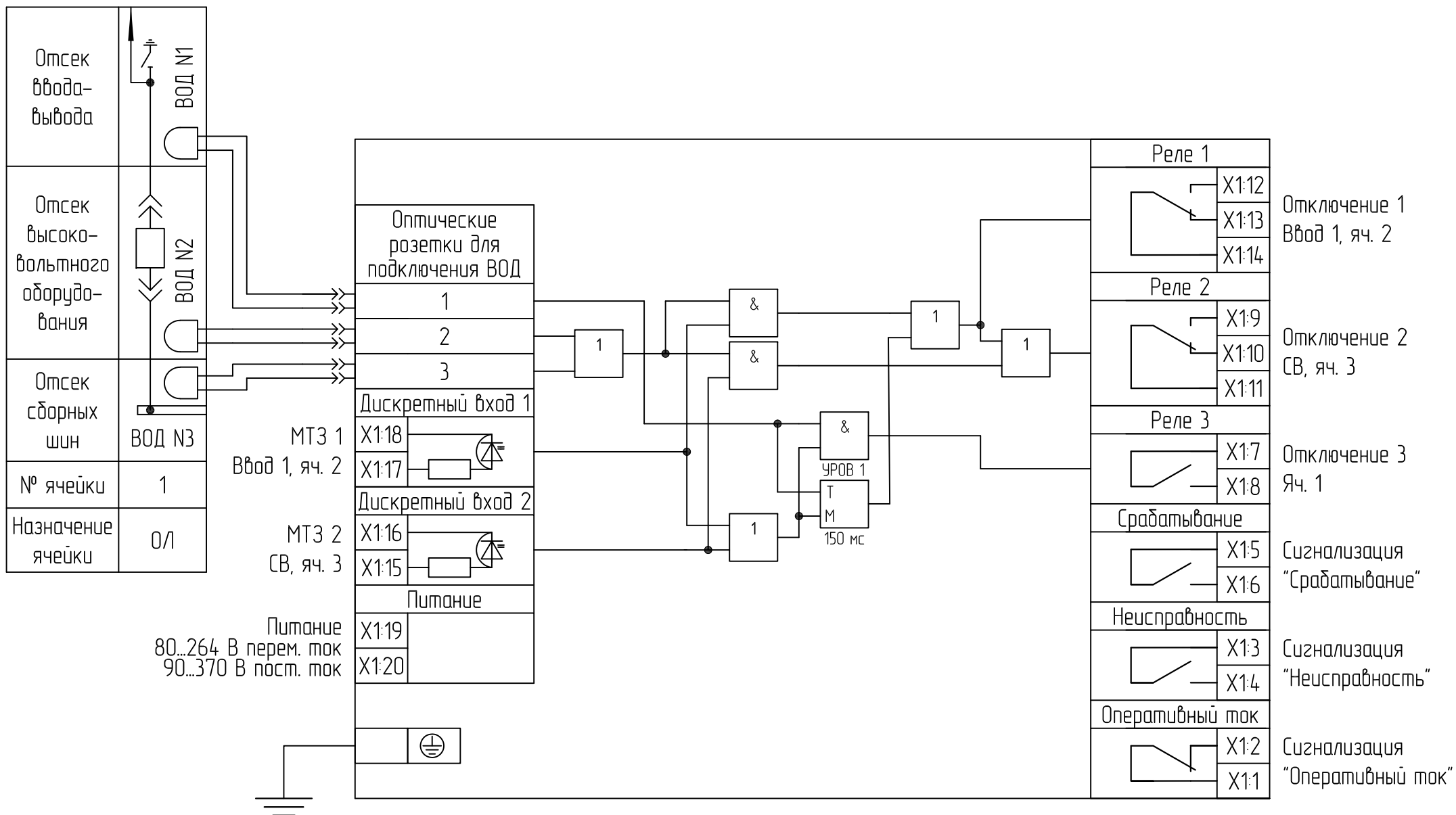
Схема подключений и логика работы УДЗ "ПРОЭЛ-МИНИ"
