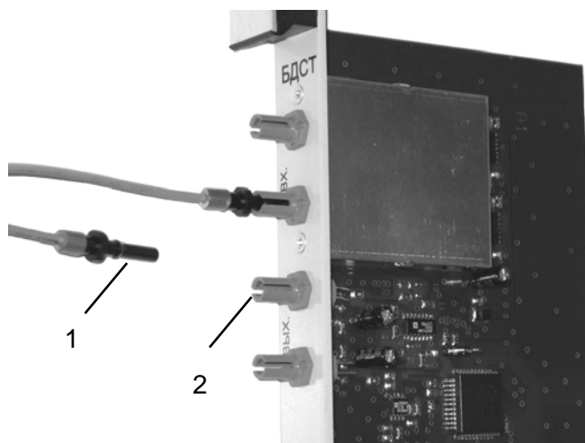
Рис. 1.8. Пластиковый коннектор: 1 - вилка; 2 - розетка
