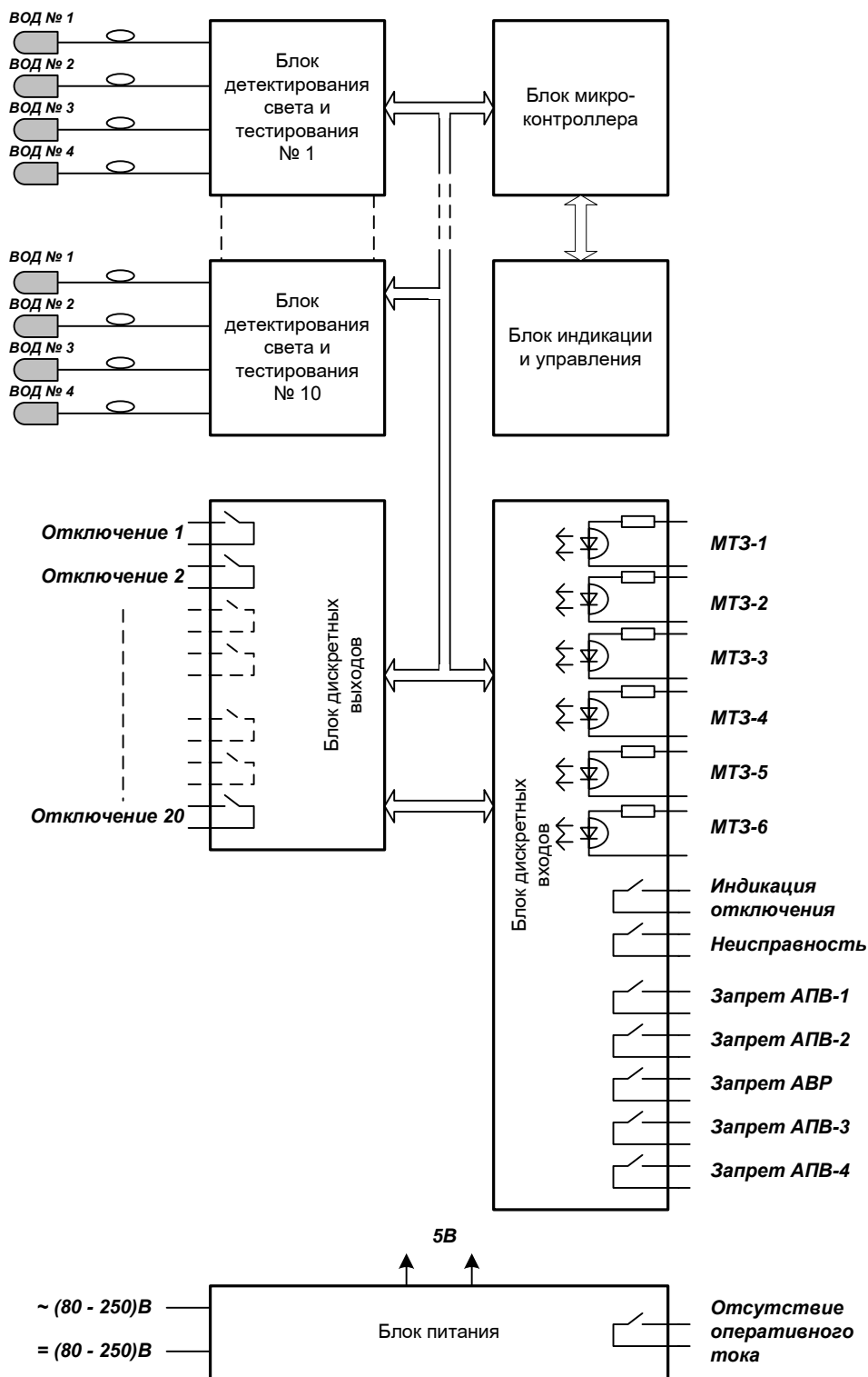
Рис.1.6. Структурная схема устройства
