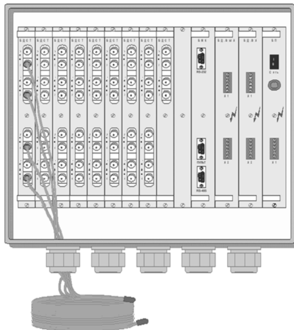
Рис. 1.4. Внутренний вид БПМ
