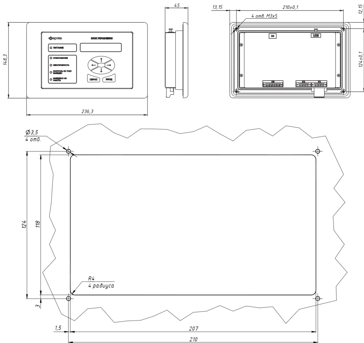
Рис. 1.14 Габаритный чертеж БУП и чертеж разметки для доработки панели.
