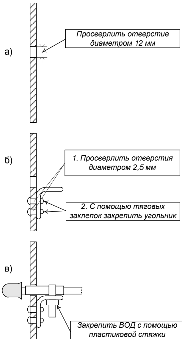
Рис. 2.4 Установка ВОД в отсеке ячейки.
