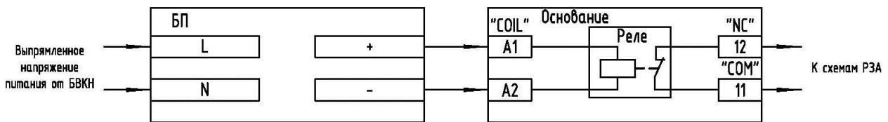
Рис. 1.37. Схема подключения реле формирования сигнала отсутствия оперативного тока при использовании нормально замкнутого контакта
