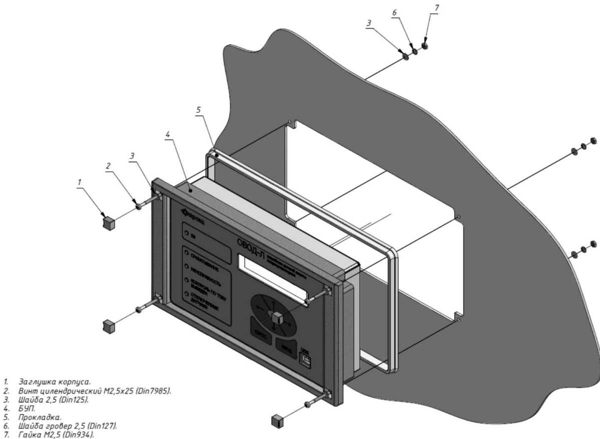
Рис. 2.4. Установка БУП
