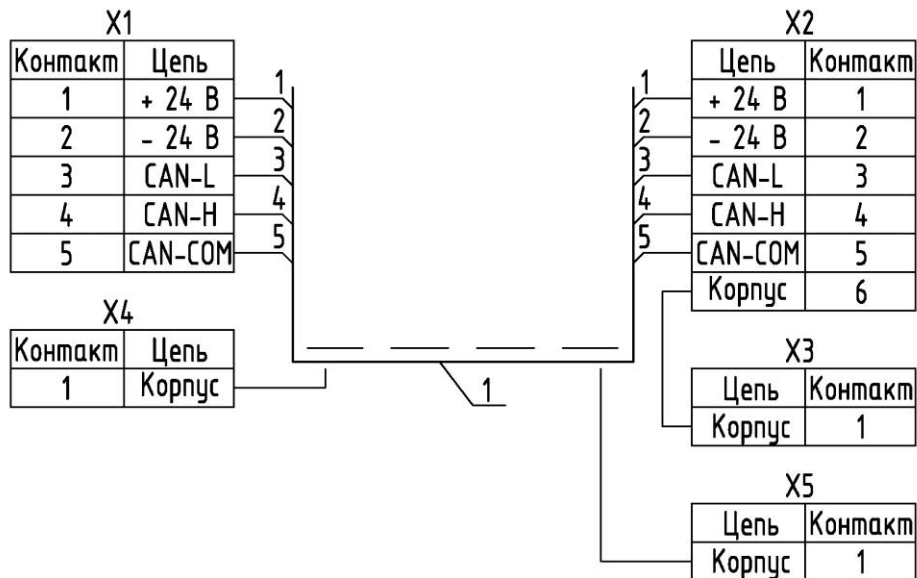
Рис. 2.10. Схема электрическая принципиальная соединительного кабеля Тип 3
