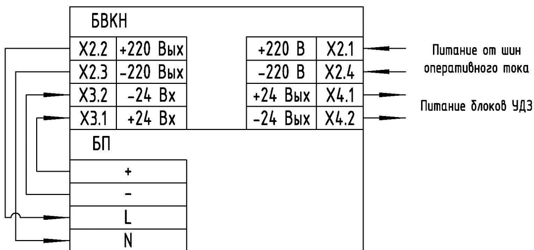
Рис. 1.36. Схема подключения БВКН и БП
