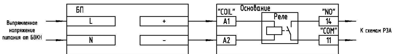
Рис. 1.38. Схема подключения реле формирования сигнала отсутствия оперативного тока при использовании нормально разомкнутого контакта
